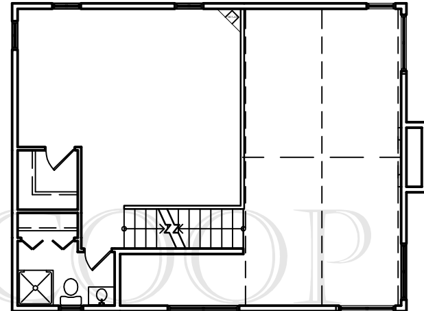
LOFT PLAN
